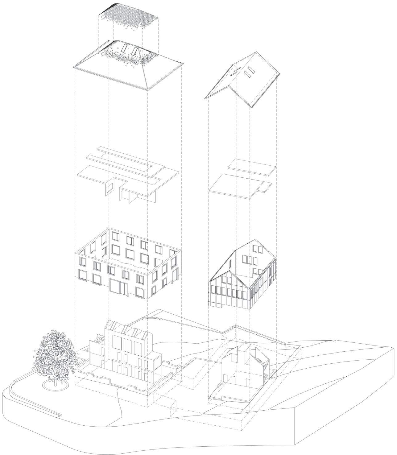
Explosionsschema
